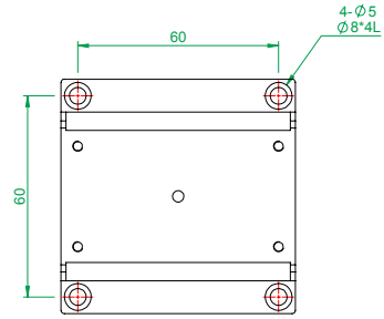
MX(Y)70-S系列 底座安裝孔尺寸
