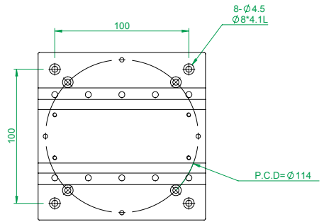
MX(Y)L125-A系列 底座安裝孔尺寸
