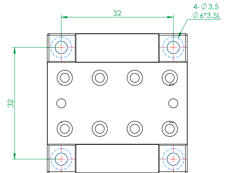
MX(Y)40-A系列 底座安裝孔尺寸
