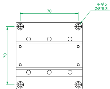
MX(Y)80-A-18系列 底座安裝孔尺寸
