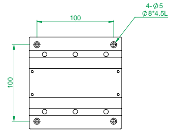
MX(Y)120-A-18系列 底座安裝孔尺寸
