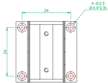
MX(Y)30-S-28系列 底座安裝孔尺寸
